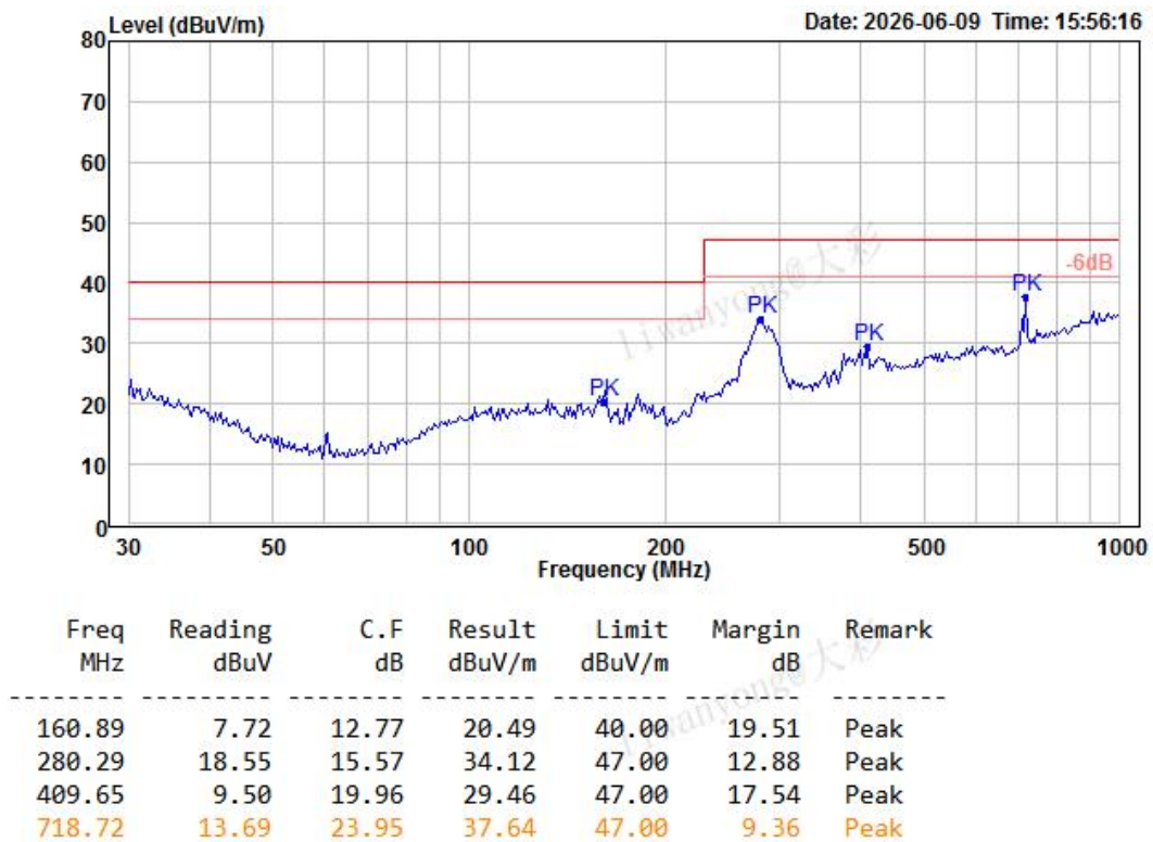
图 6-6 辐射测试水平方向
