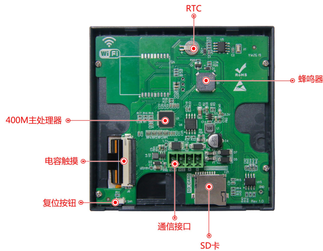
图 1-2 硬件配置图
