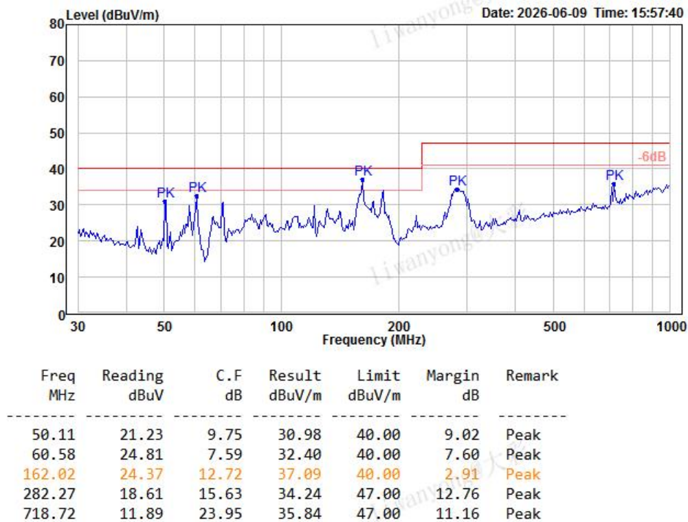
图 6-7 辐射测试垂直方向
