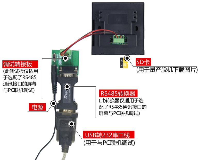
图 1-3 调试工具图
